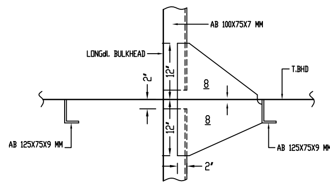
A-A SECTION
