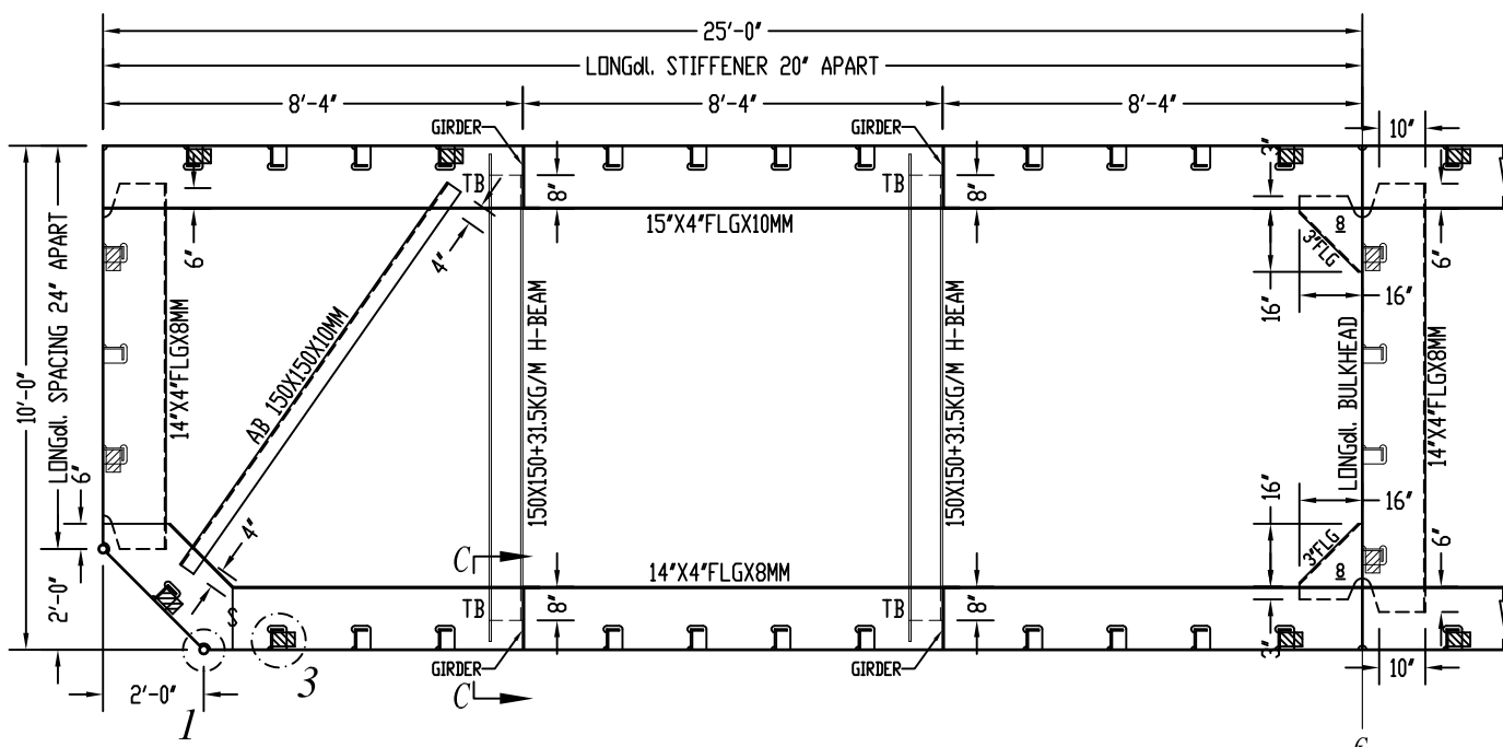
TRANSVERSAL WEB SECTION(TYP)
